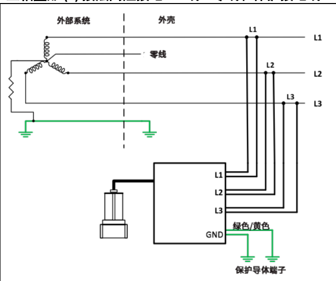
三相星形 (Y) 接法高阻接地：3 线 + 零线和保护接地线
