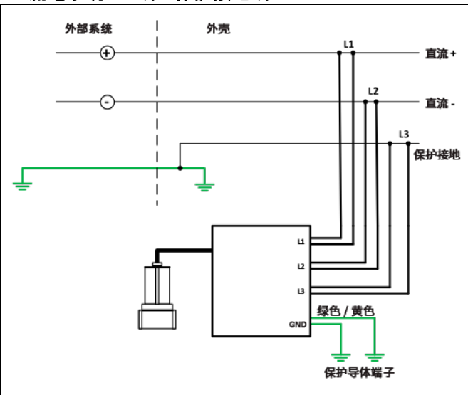
直流电系统：2 线 + 保护接地线
