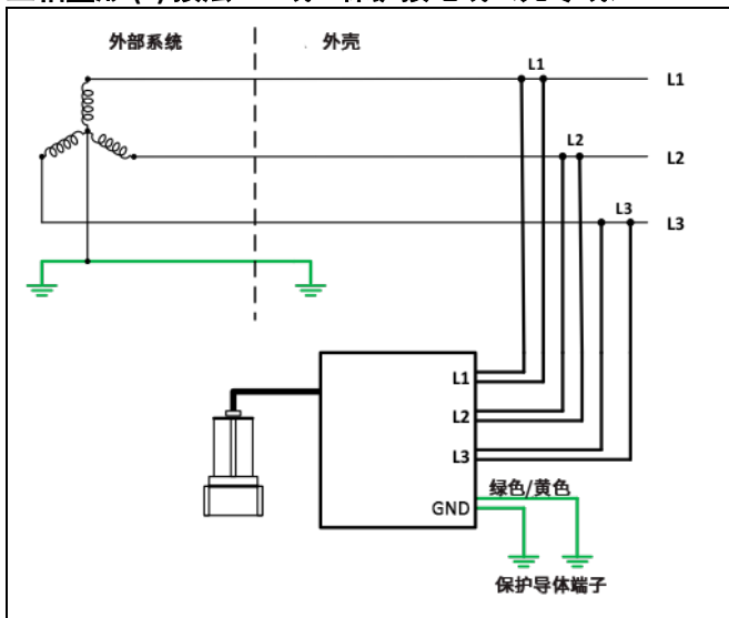
三相星形 (Y) 接法：3 线 + 保护接地线（无零线）
