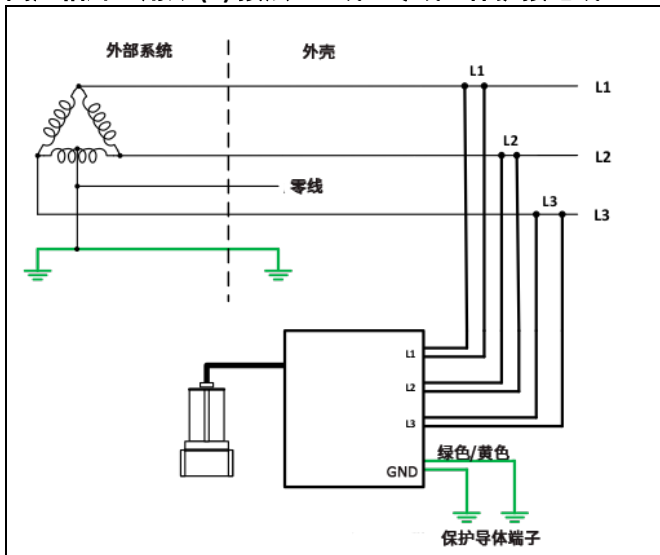
高压相脚三角形 (Δ) 接法：3 线 + 零线 + 保护接地线
