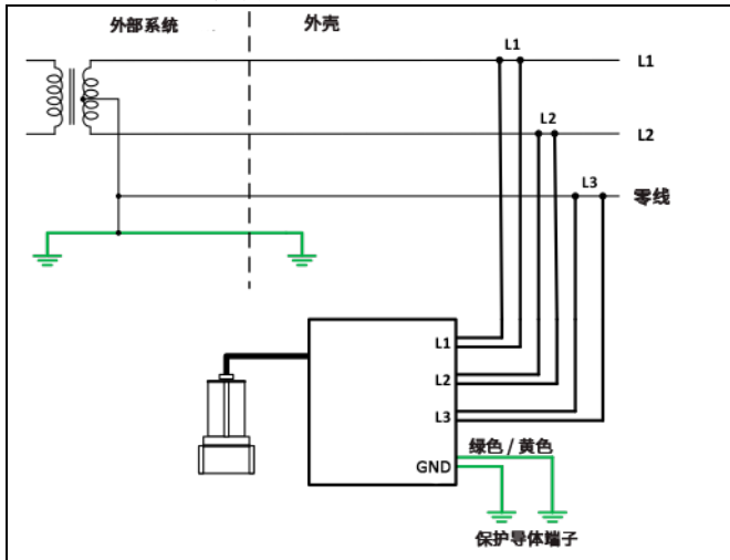
高压相脚三角形 (Δ) 接法：3 线 + 零线 + 保护接地线
