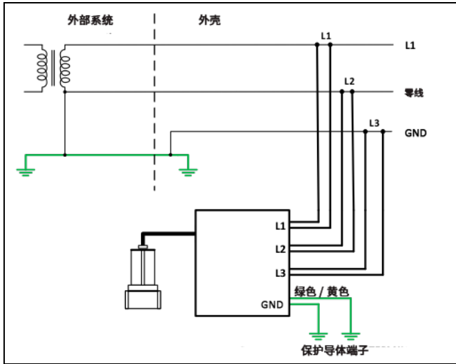
单相：2 线 + 保护接地线
