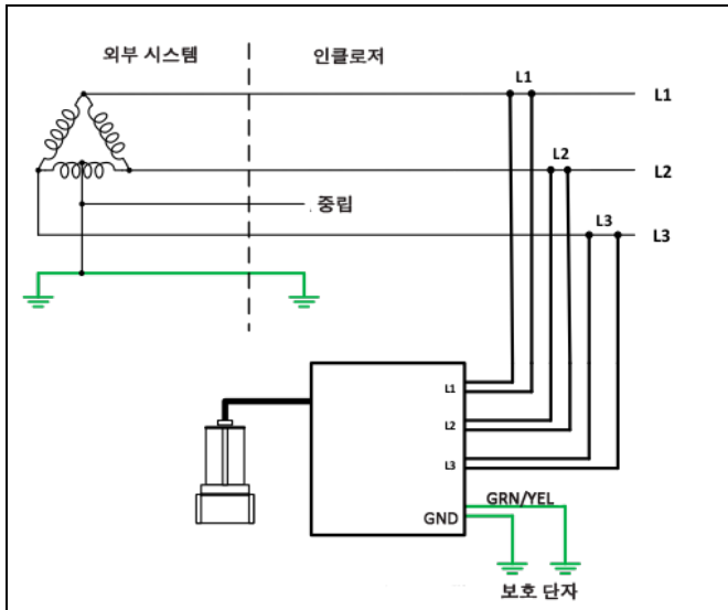
하이 레그 DELTA: 3선 + 중립 + PE
