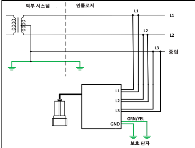
하이 레그 DELTA: 3선 + 중립 + PE
