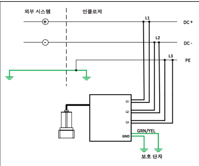
DC 시스템: 2선 + PE
